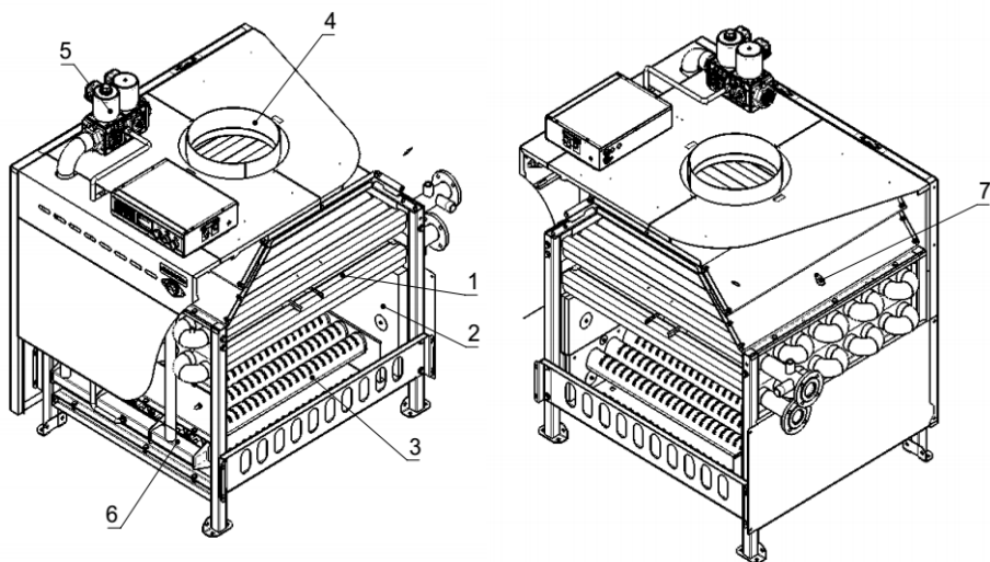
Рисунок 2. Общий вид котла RSA
