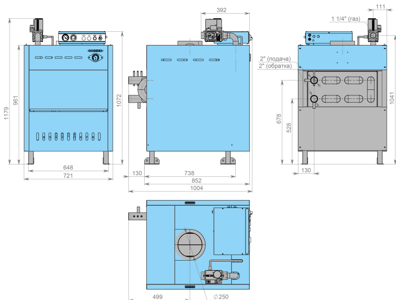
Рисунок 1. Габаритно-присоединительные размеры котла RSA120
