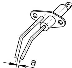
Рисунок 10. Электрод розжига
