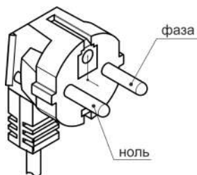
Рисунок 11. Вилка пульта управления котла
