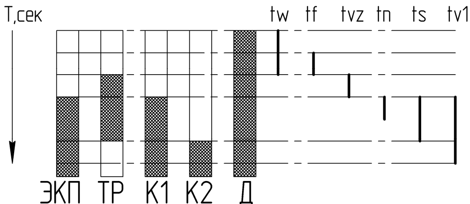
Рисунок 7. Контроллер розжига DKG 972
