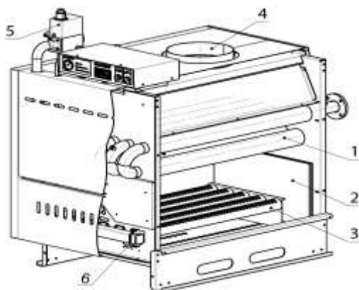
Рисунок 4. Устройство котла
