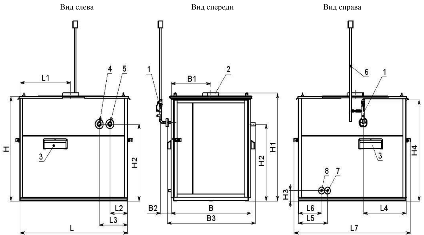
Рисунок 1. Габаритно-присоединительные размеры котлов RS-H40, RS-H60, RS-H80, RS-H100, RS-H150, RS-H200, RS-H300 (см. Таблицу 2)
