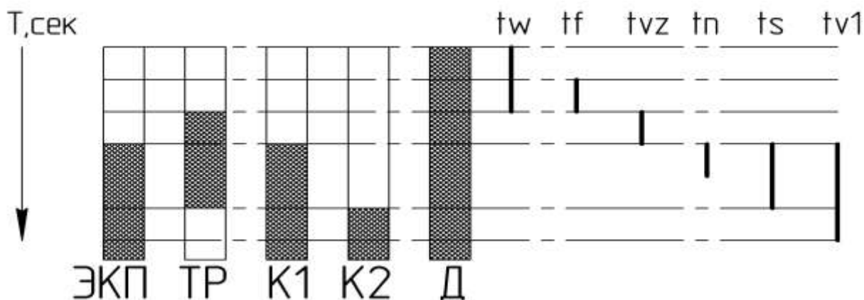
ЭКП - электрод контроля пламени, Тр - трансформатор розжига, К1 - газовый клапан растопочной горелки, К2 - газовый клапан малого горения, Д - дымосос (наличие зависит от комплектации котла).
