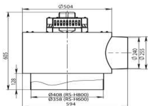
Рисунок 8. Габаритно-присоединительные размеры дымососа
