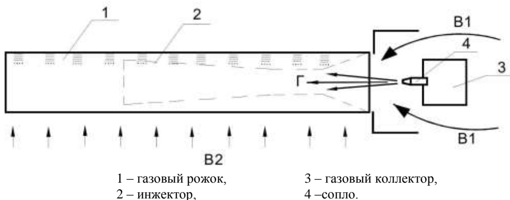
Рисунок 6. Устройство газовой горелки (вид сбоку)
