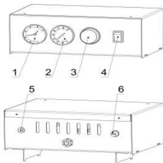
Рисунок 10. Пульт управления для котлов RSH40, RSH60
