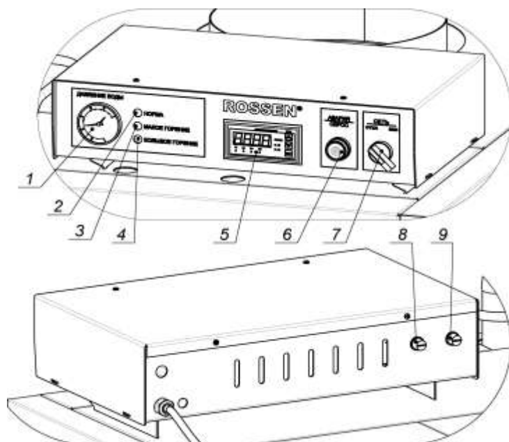
Рисунок 12. Пульт управления для котлов RSH150, RSH200, RSH300, RSH400, RSH500
