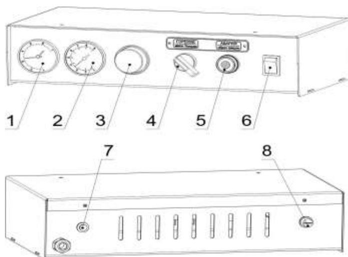
Рисунок 10. Пульт управления для котлов RSH40, RSH60
