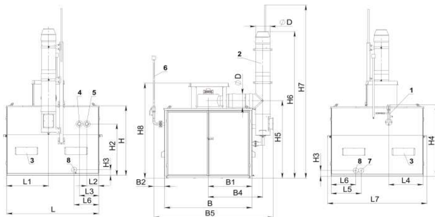
Рисунок 3. Габаритно-присоединительные размеры с дымососом для котлов RS-H200, RS-H300, RS-H 400
