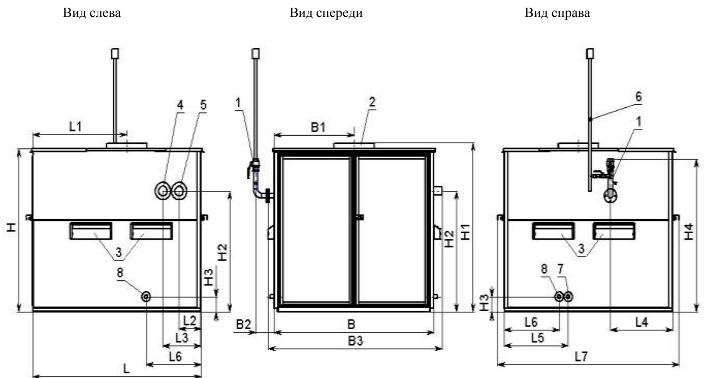
Рисунок 2. Габаритно-присоединительные размеры котлов RS-H400, RS-H500 (см. Таблицу 2)
